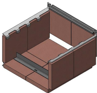
Area di combustione inferiore - tappo di chiusura smontato
