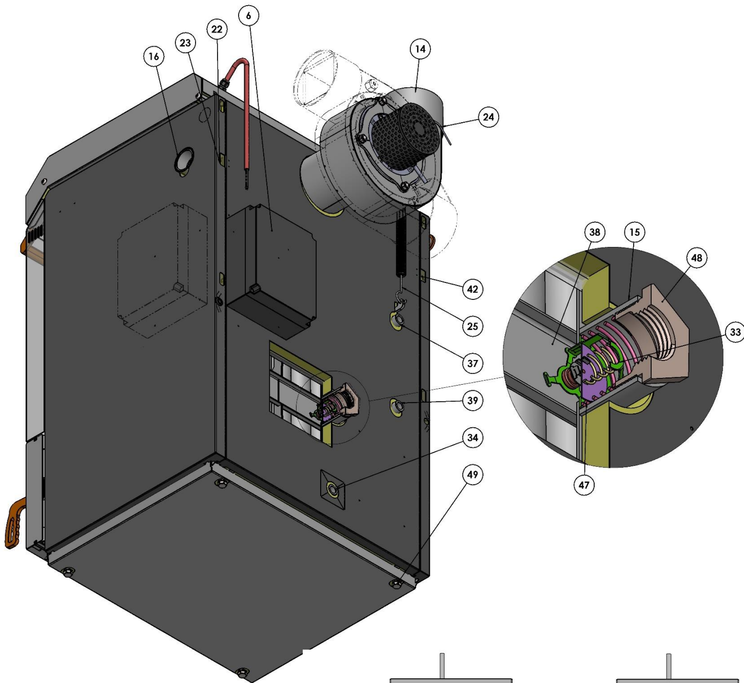
Schema della caldaia - vista posteriore
