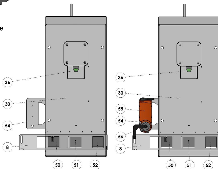
Schema della caldaia - dettaglio della ventilazione
